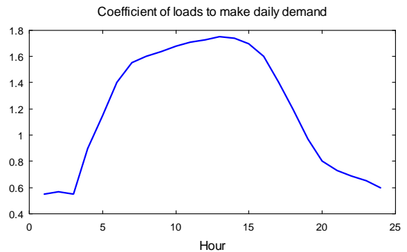
شکل ۳: ضریب بار شبکه (به جز بار شارژ خودروها) در ساعات مختلف
